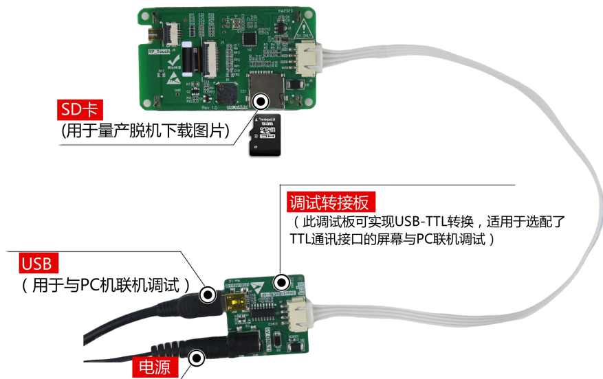
图 1-4 调试工具图
