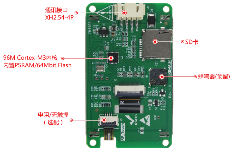
图 1-3 硬件配置图
